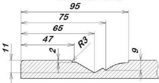
глухой рамка 65 мм
