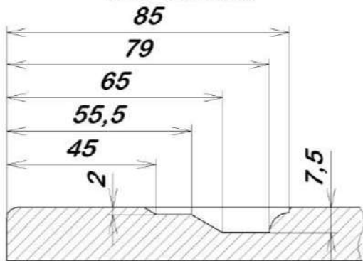
глухой рамка 65 мм
